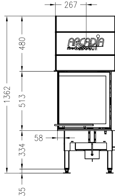
Vorderansicht M~1:20
