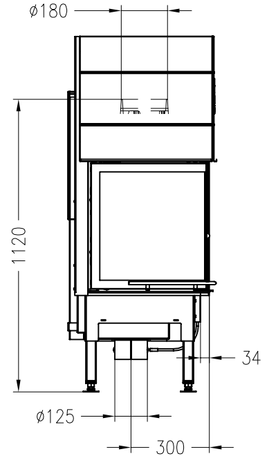
Seitenansicht M~1:20
