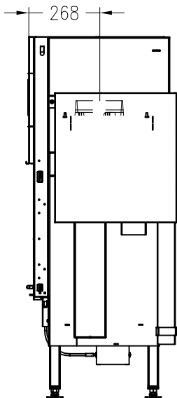
Seitenansicht M~1:20
